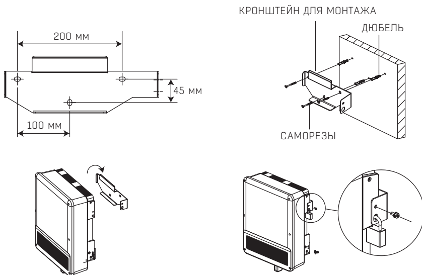
Рисунок 3.4.4 Инструкция по креплению инвертора на поверхность
