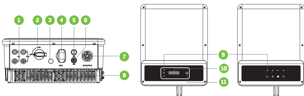
Рисунок 2.3.1 Схема инвертора
